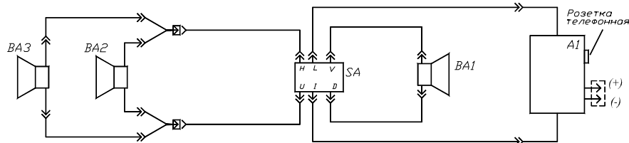
Рисунок 1.1 – Схема соединений.
