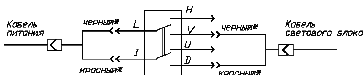
Рисунок 2.7 – Рекомендуемая схема подключения к переключателю П147 (*цвета держателей)
